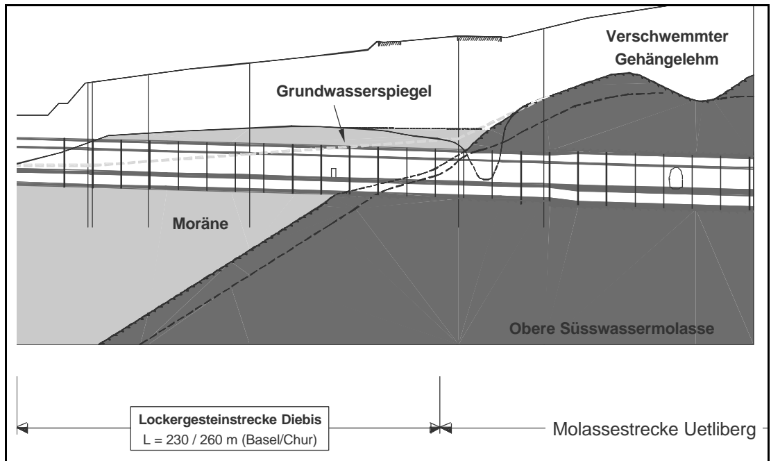
Geologisches Längenprofil Diebis (Lockergesteinsvortrieb im Gange)
