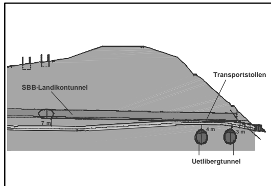
Längsschnitt SBB-Tunnel
