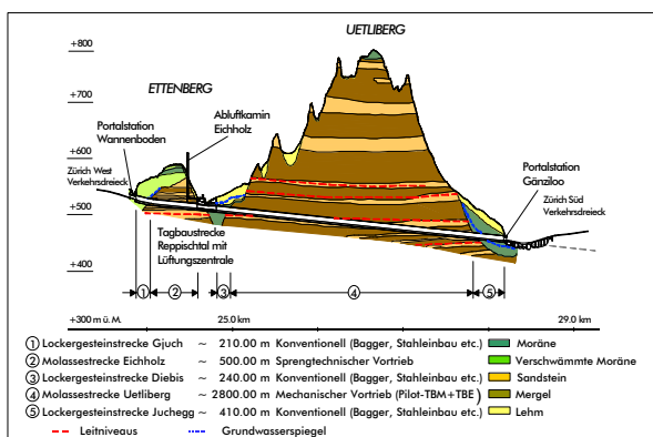
Geologisches Längenprofil und Vortriebsverfahren
